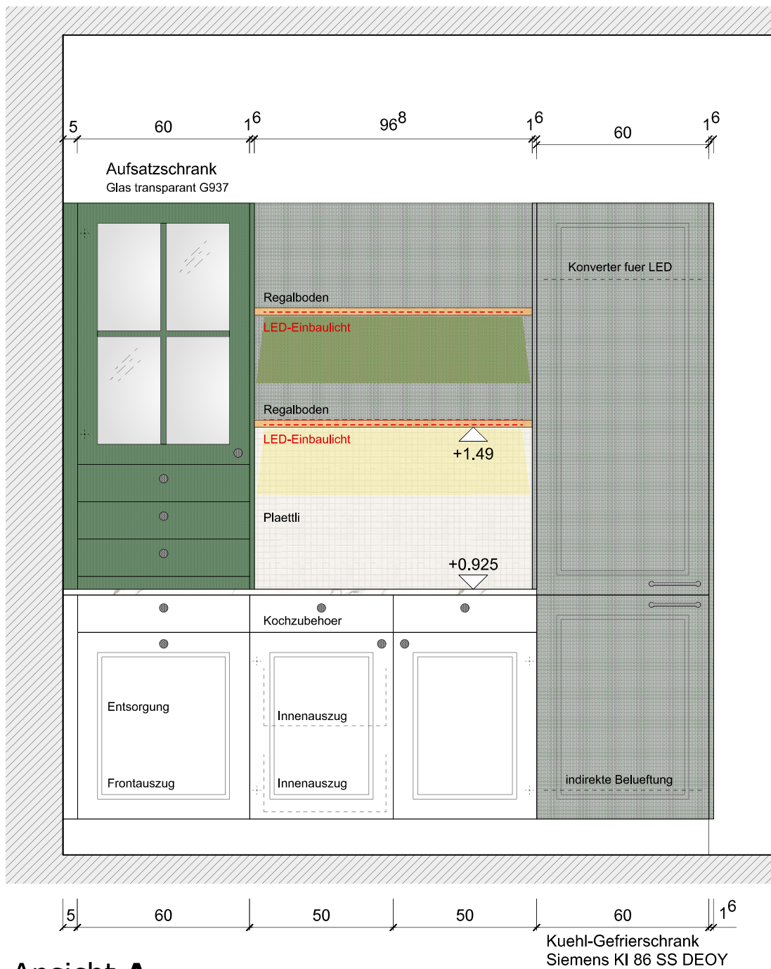
Ansicht A
