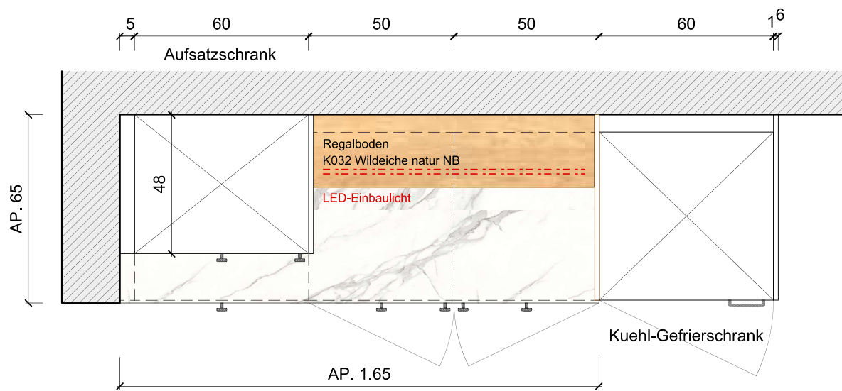
Grundriss
